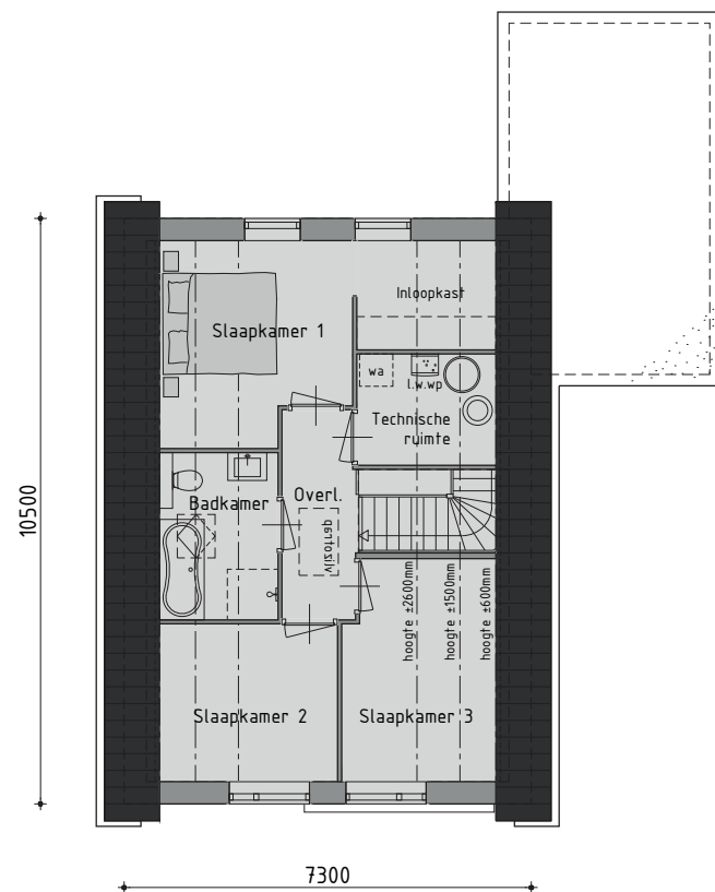
1e VERDIEPING
