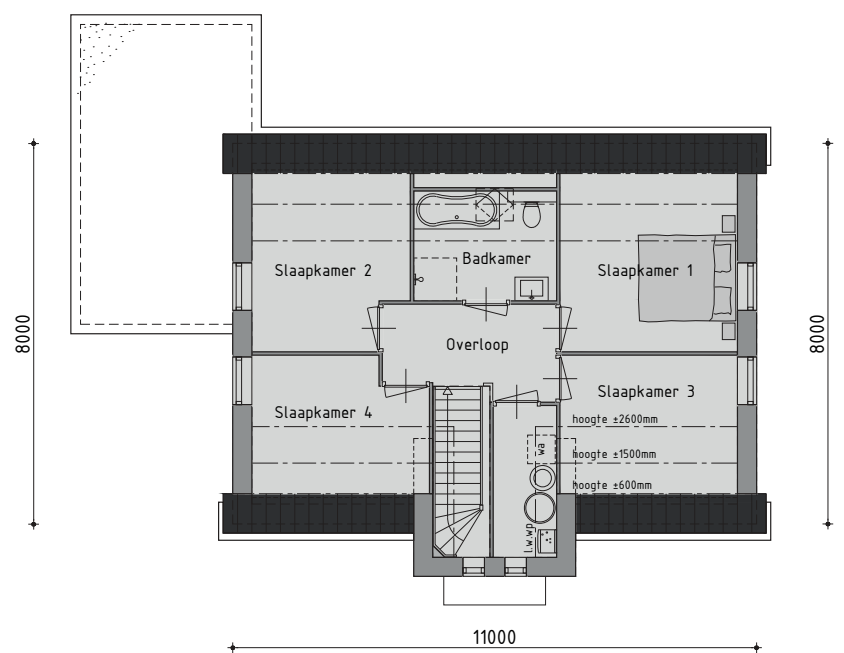
1 e VERDIEPING
