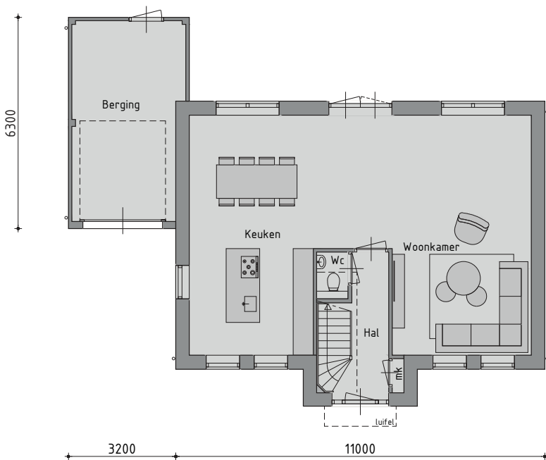
BEGANE GROND
