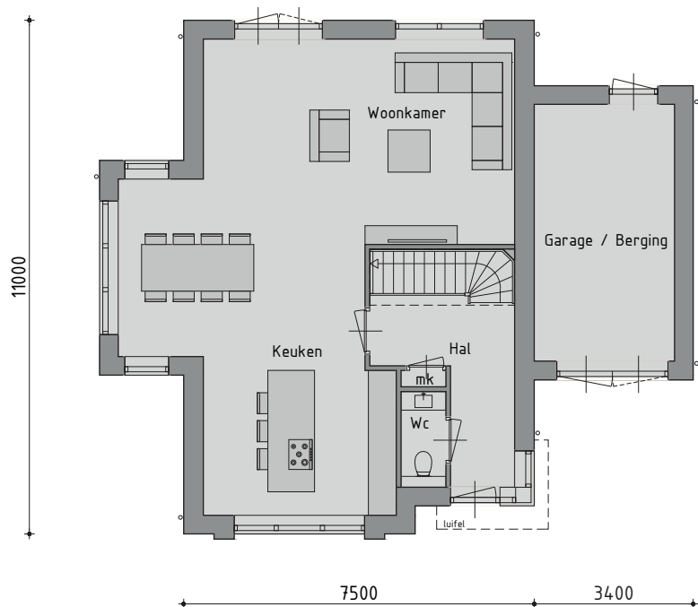
BEGANE GROND
