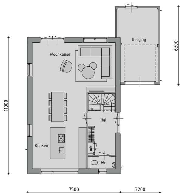
BEGANE GROND
