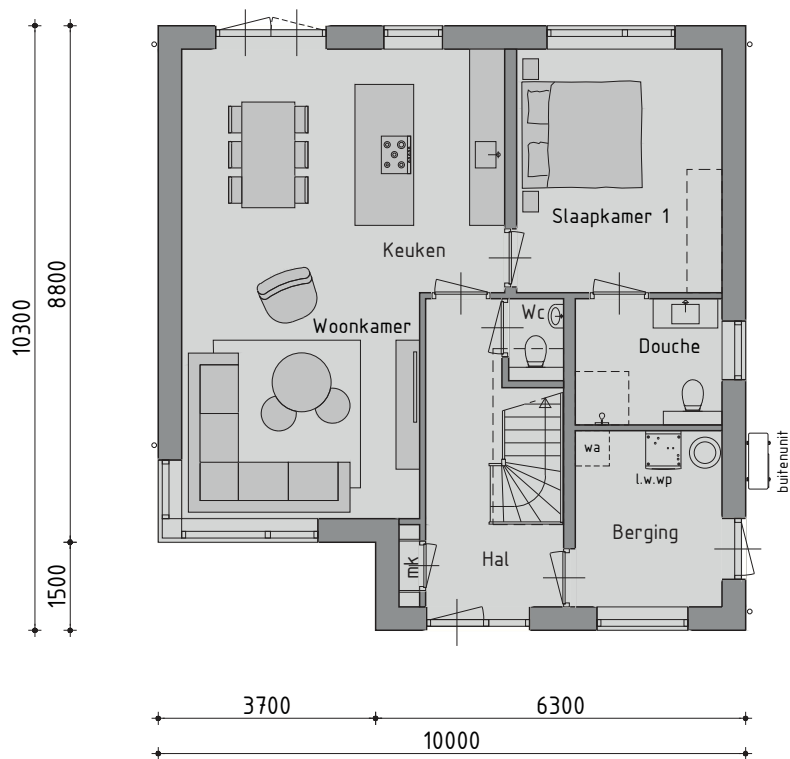
BEGANE GROND
