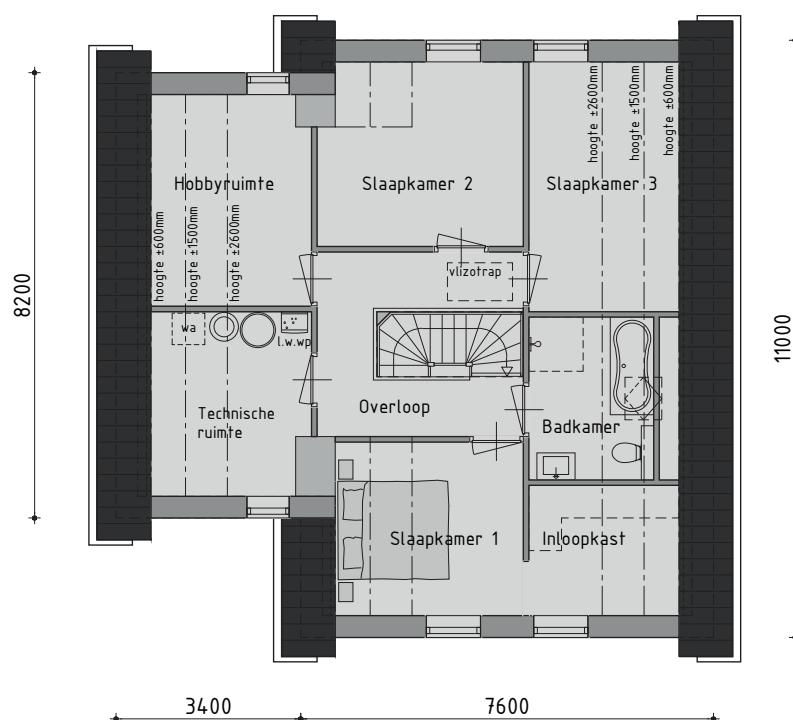
1e VERDIEPING
