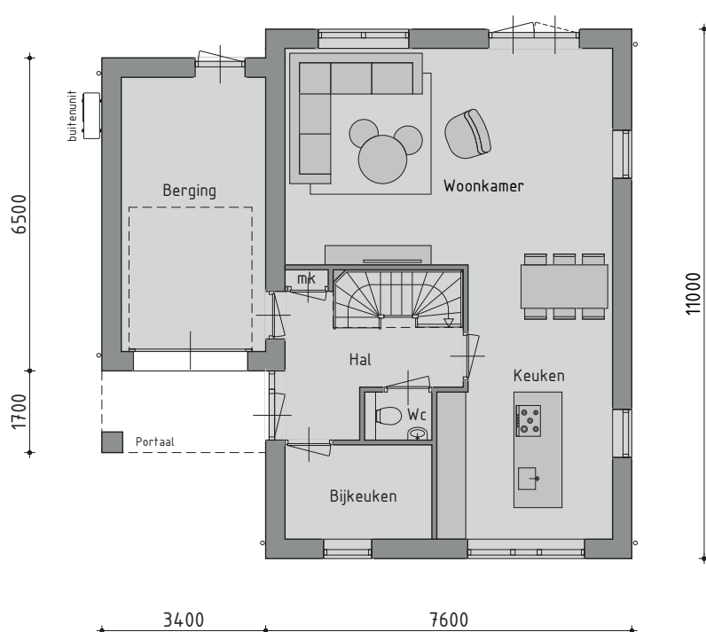
BEGANE GROND
