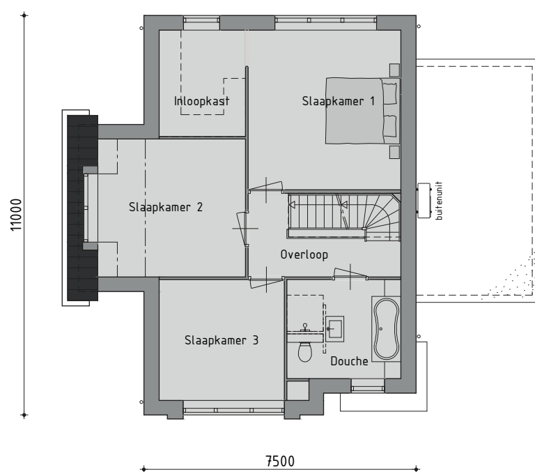
1 e VERDIEPING
