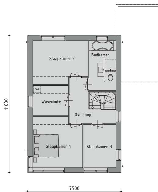
1 e VERDIEPING
