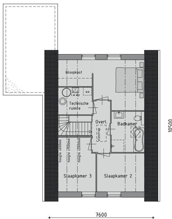
1e VERDIEPING
