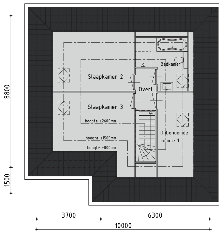
1 e VERDIEPING
